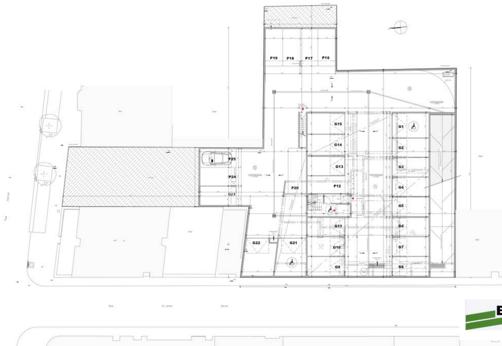
PLAN DE SOUS-SOL Ech 1/200
